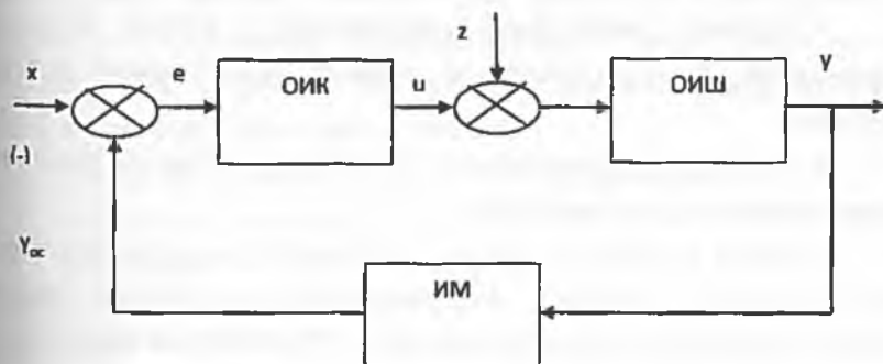
Расми.3.6. Схемати структурии система бастаи идоранамой
