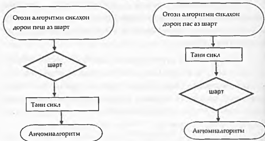
Расми 2.16. Алгоритмҳои даврӣ ё сиклӣ
