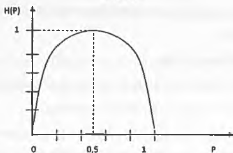
Расми 3.9. Вобастагии энтропия аз эҳтимоли яке аз ду ҳолат.
