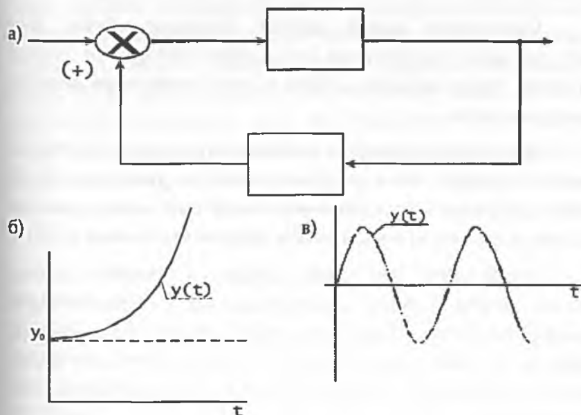
Рис. 3.8. Нақшаи структурии системаи дорои алоқаи баръакси мусбат:
