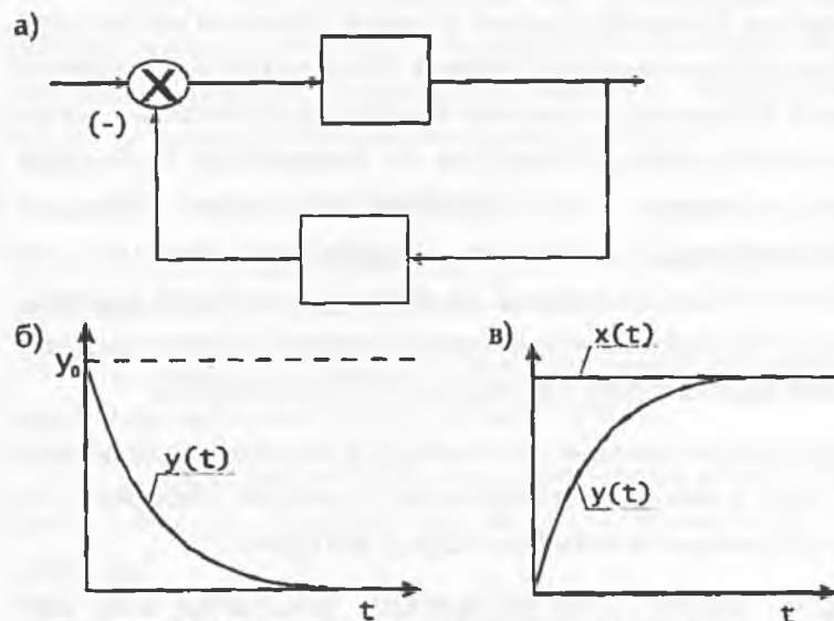
Расми 3.7. Нақшаи структурии системаи дорои алоқаи манфии баръакс:
