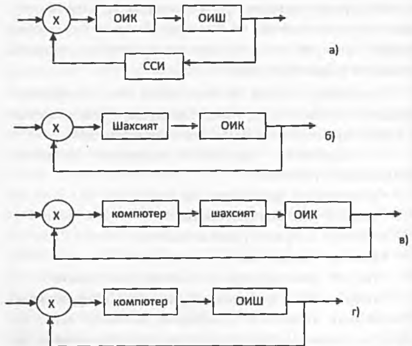
Расми.3.2. Нақшаи структурии системаи идоранамоӣ
